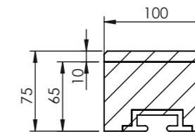
SEZIONE A-A
